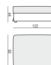
FOOTSTOOL 122x92
